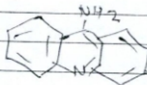
aminoacridine.
