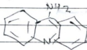
aminoacridine.
